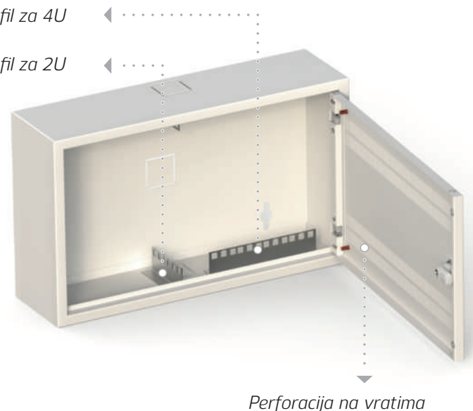
Izgled ormana RKL 4/2NH
