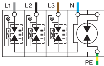
OVR T1+2 3N 15 255-7
